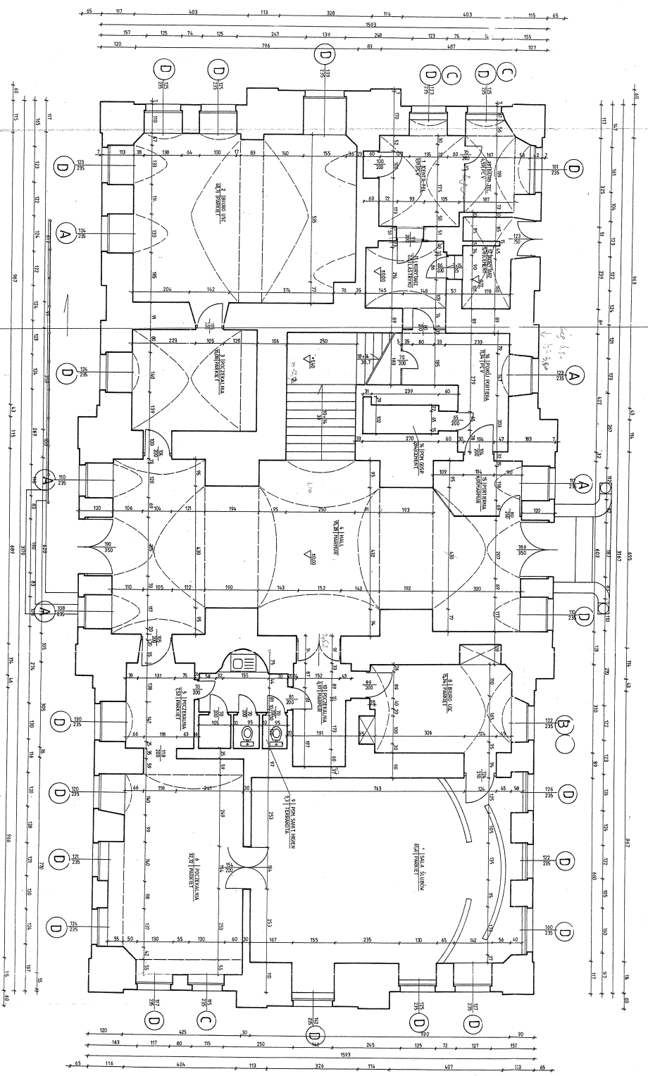
RZUT PARTERU
