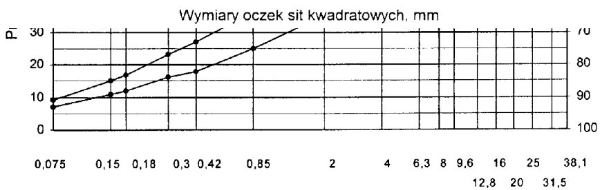
Rys. 7. Krzywe graniczne uziarnienia mieszanki mineralnej BA od 0 do 12,8 mm do warstwy
